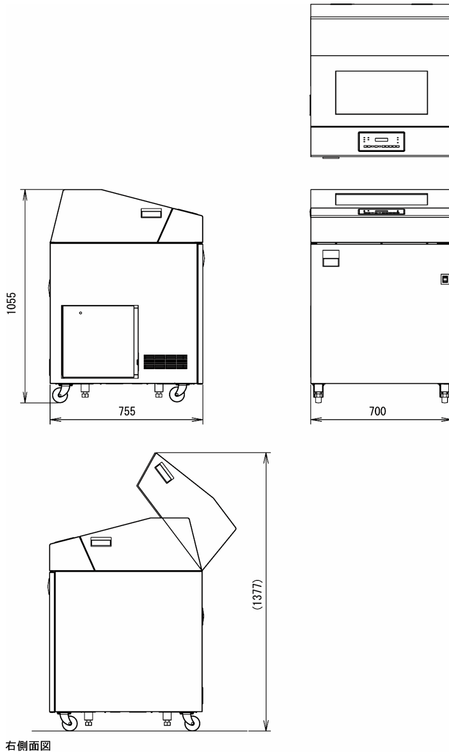
図 15 外形寸法
